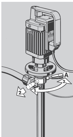
Модель насоса - RE- Niro / Тръба на помпата RE SS / Брашъл помпей RE Niro рис. / Фиг. / Fig. 6
